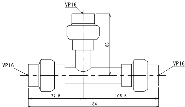
ISO継手寸法(コンパ 外エノンタイプ)
